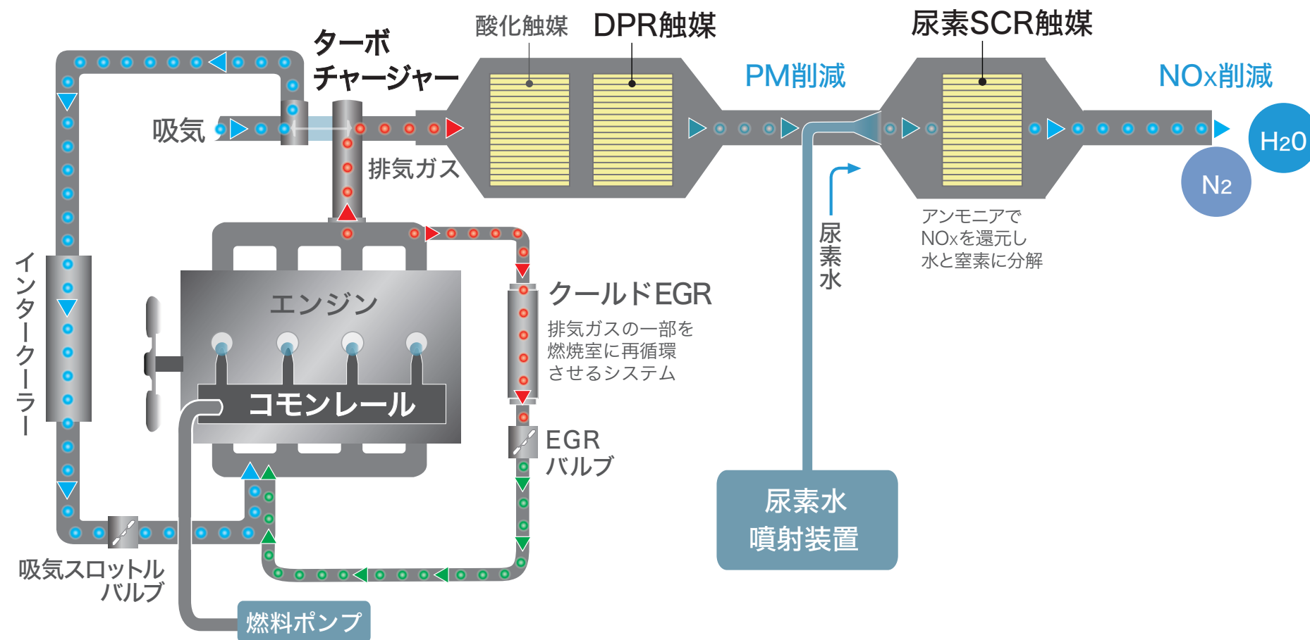
1GD-FTVエンジン システム図
